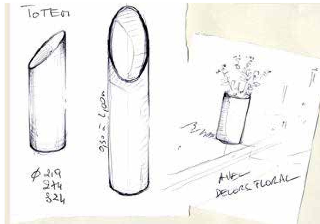
ci-contre : Totem «bienvenue» végétalisé tube en acier rouillé, gravé au laser, équipé d'un bac à fleur dimensions : 1100 mm x Ø 324 mm
